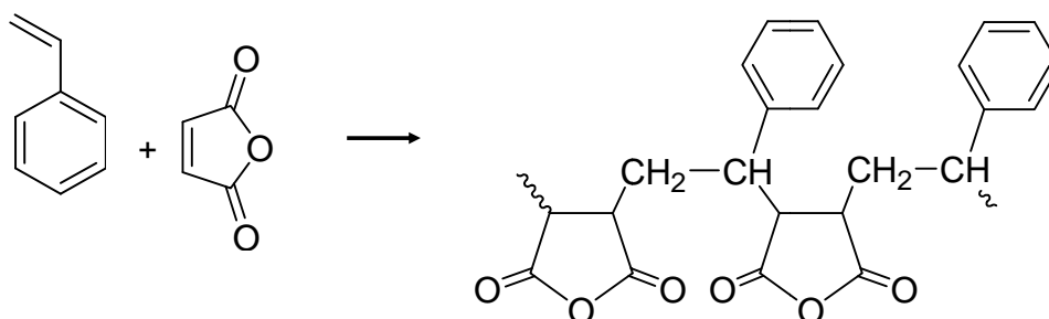
Copolymère styrène – alt – anhydride maléique
